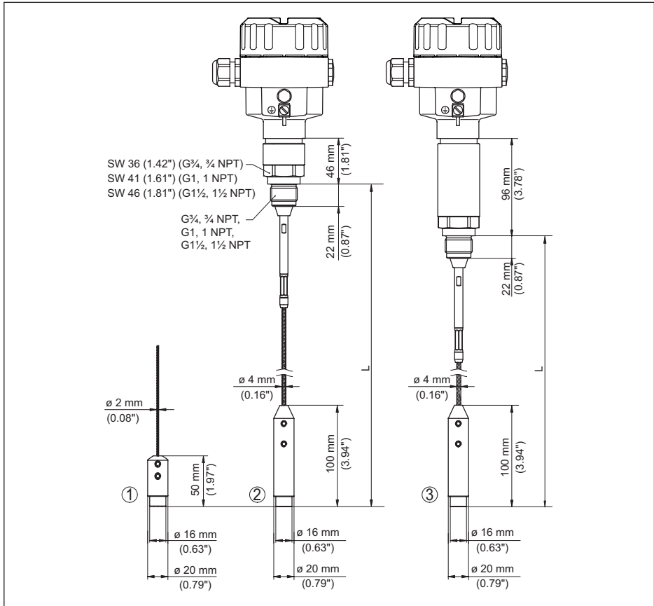
Abb. 42: NivoGuide 8100, Gewindeausführung mit Straffgewicht (alle Straffgewichte mit Gewinde M8 für Ringschraube)
