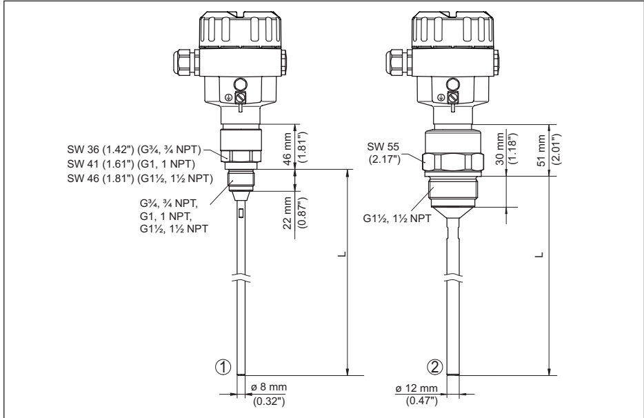
Abb. 43: NivoGuide 8100, Gewindeausführung
