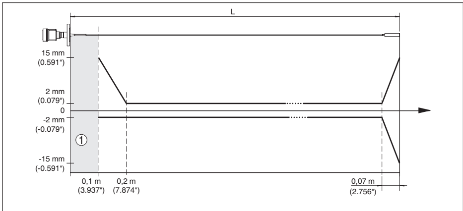
Abb. 36: Messabweichung NivoGuide 8100 in Seilausführung ( \varnothing 4 mm/0.157 in, PFA-beschichtet) in Medium Wasser
