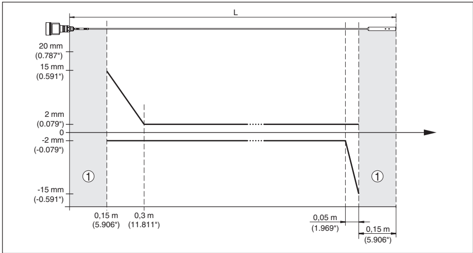
Abb. 35: Messabweichung NivoGuide 8100 in Seilausführung ( \varnothing 4 mm/0.157 in), in Medium Öl
