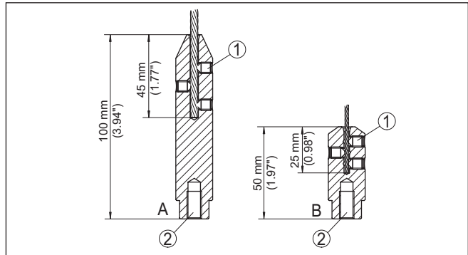
Abb. 29: Seilmesssonde kürzen
