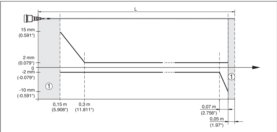
Abb. 32: Messabweichung NivoGuide 8100 in Stabausführung in Medium Öl
