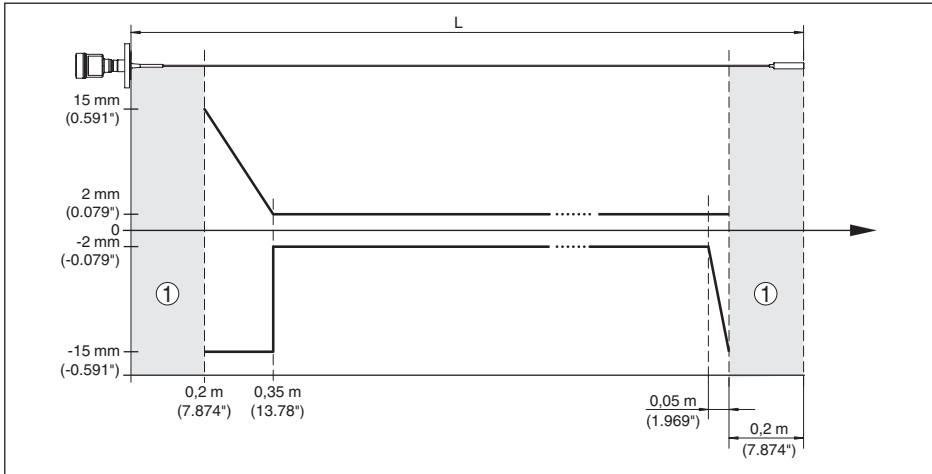
Abb. 37: Messabweichung NivoGuide 8100 in Seilausführung ( \varnothing 4 mm/0.157 in, PFA-beschichtet) in Medium Öl 1 Blockdistanz (in diesem Bereich ist keine Messung möglich) L Sondenlänge
