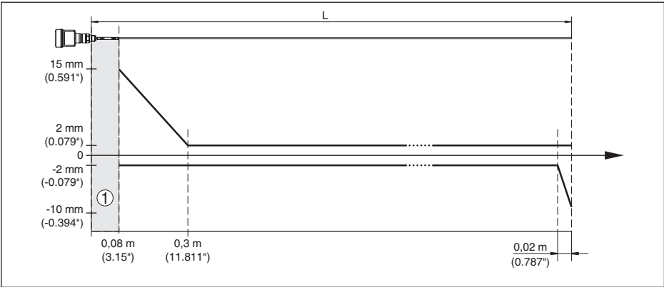
Abb. 31: Messabweichung NivoGuide 8100 in Stabausführung in Medium Wasser
