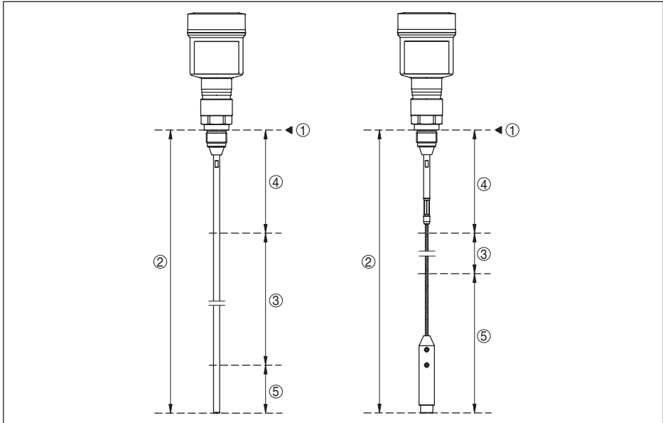
Abb. 30: Messbereiche - NivoGuide 8100
