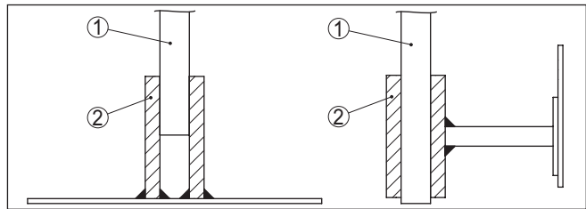
Abb. 9: Messsonde fixieren
