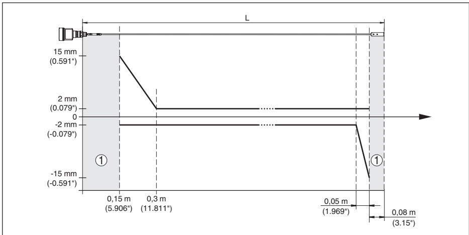
Abb. 34: Messabweichung NivoGuide 8100 in Seilausführung ( \varnothing 2 mm/0.079 in), in Medium Öl
