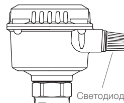
Поз.27 а, с Светодиод, установлен в кабельный ввод M20x1,5
